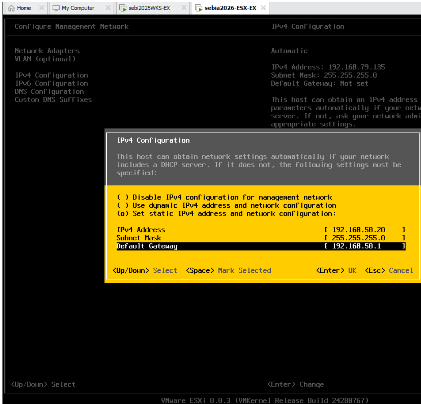
Schermafbeelding 13 — ESXi IPv4-configuratie: statisch IP 192.168.50.20, subnet .0, gateway .1
