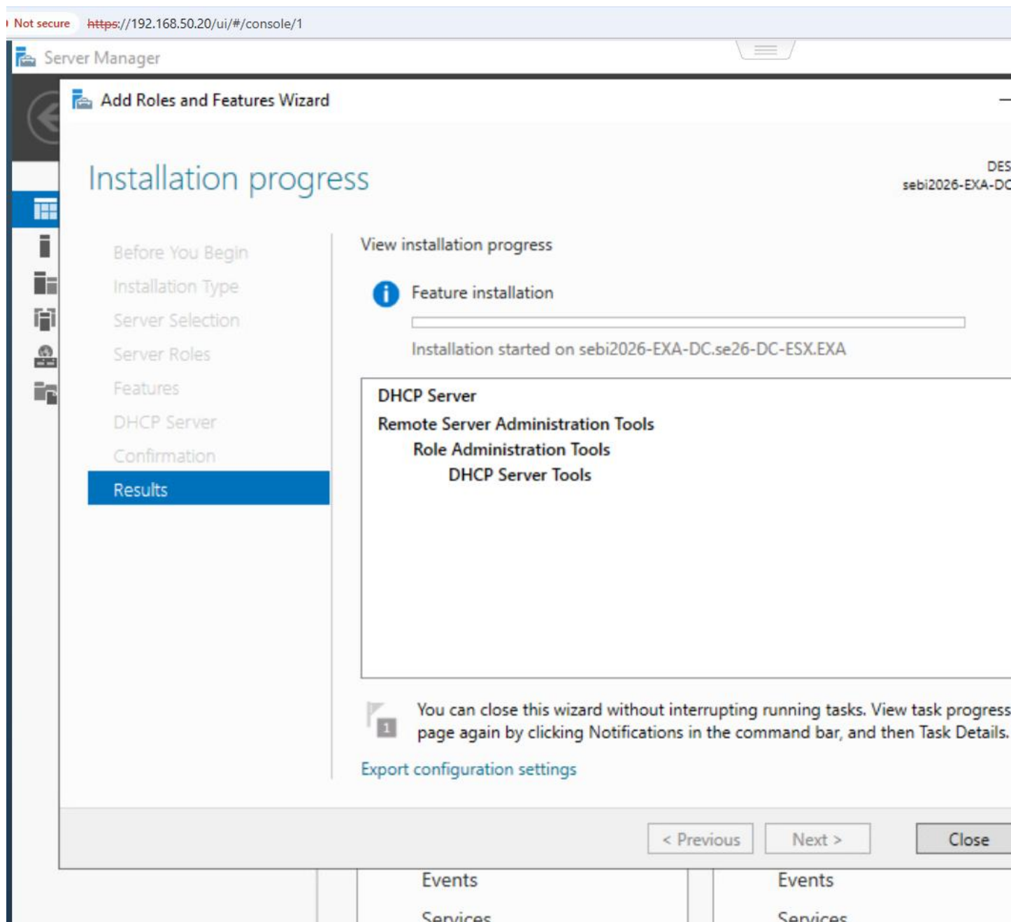
Schermafbeelding 29 — Installatie DHCP-servertools op sebi2026-EXA-DC.se26-DC-ESX.EXA in voortgang
