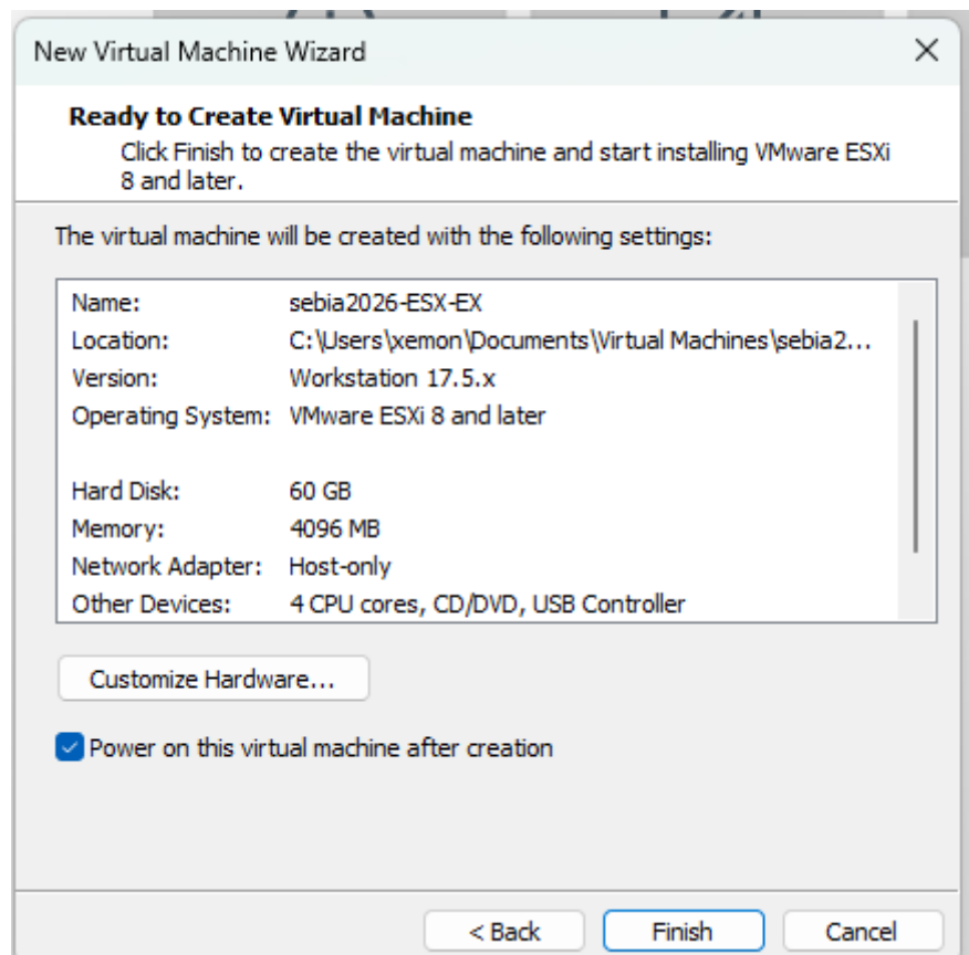
Schermafbeelding 11 — ESXi VM-aanmaak wizard: naam, 60 GB schijf, 4 GB RAM, Host-only (overzicht 1)
