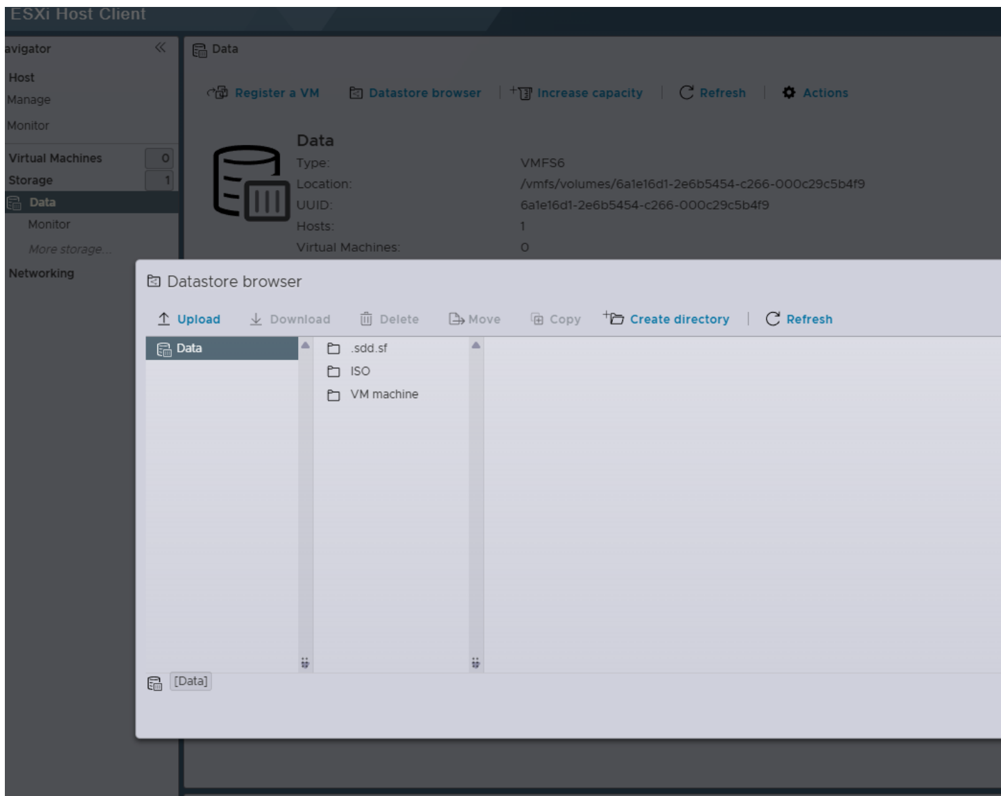
Schermafbeelding 20 — Datastore overzicht: type VMFS6, mappen .sdd.sf, ISO en VM machine zichtbaar
