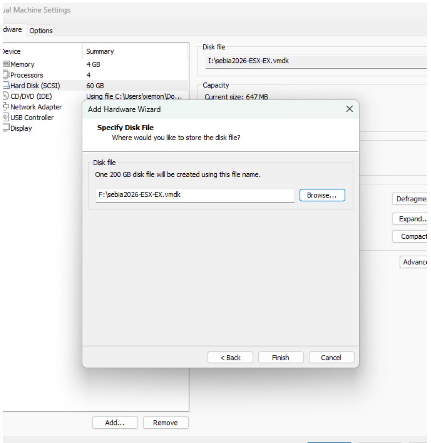
Schermafbeelding 16 — Hardware toevoegen: nieuw schijfbestand 200 GB, F:\sebia2026-ESX-EX.vmdk
