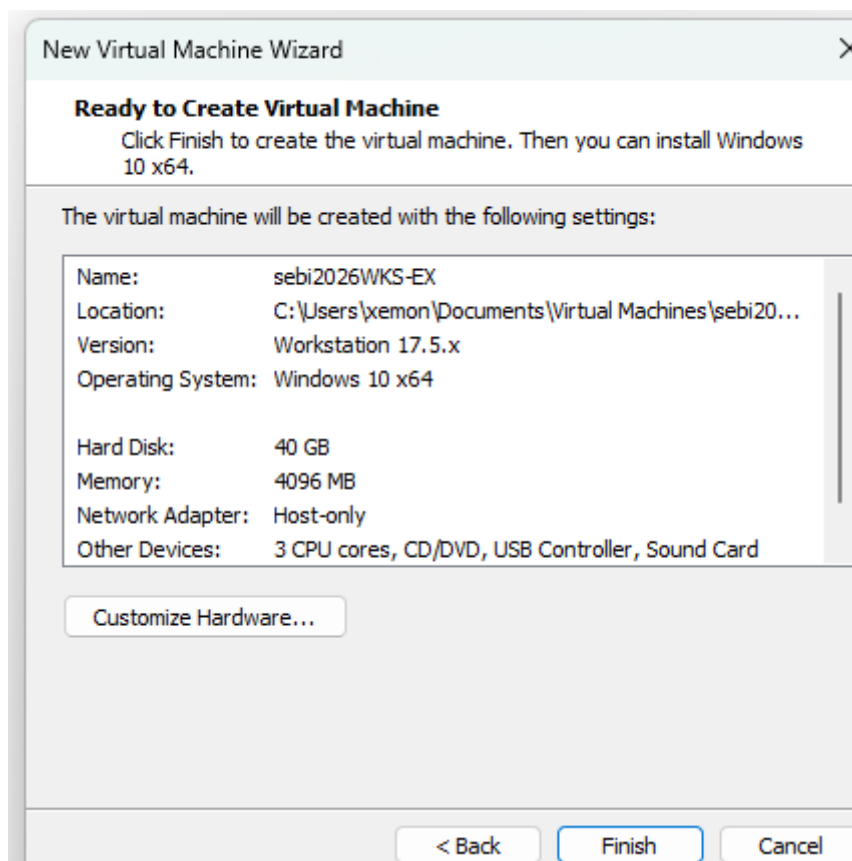
Schermafbeelding 1 — VM-aanmaak wizard: naam, schijf, netwerk en RAM (overzicht 1)
