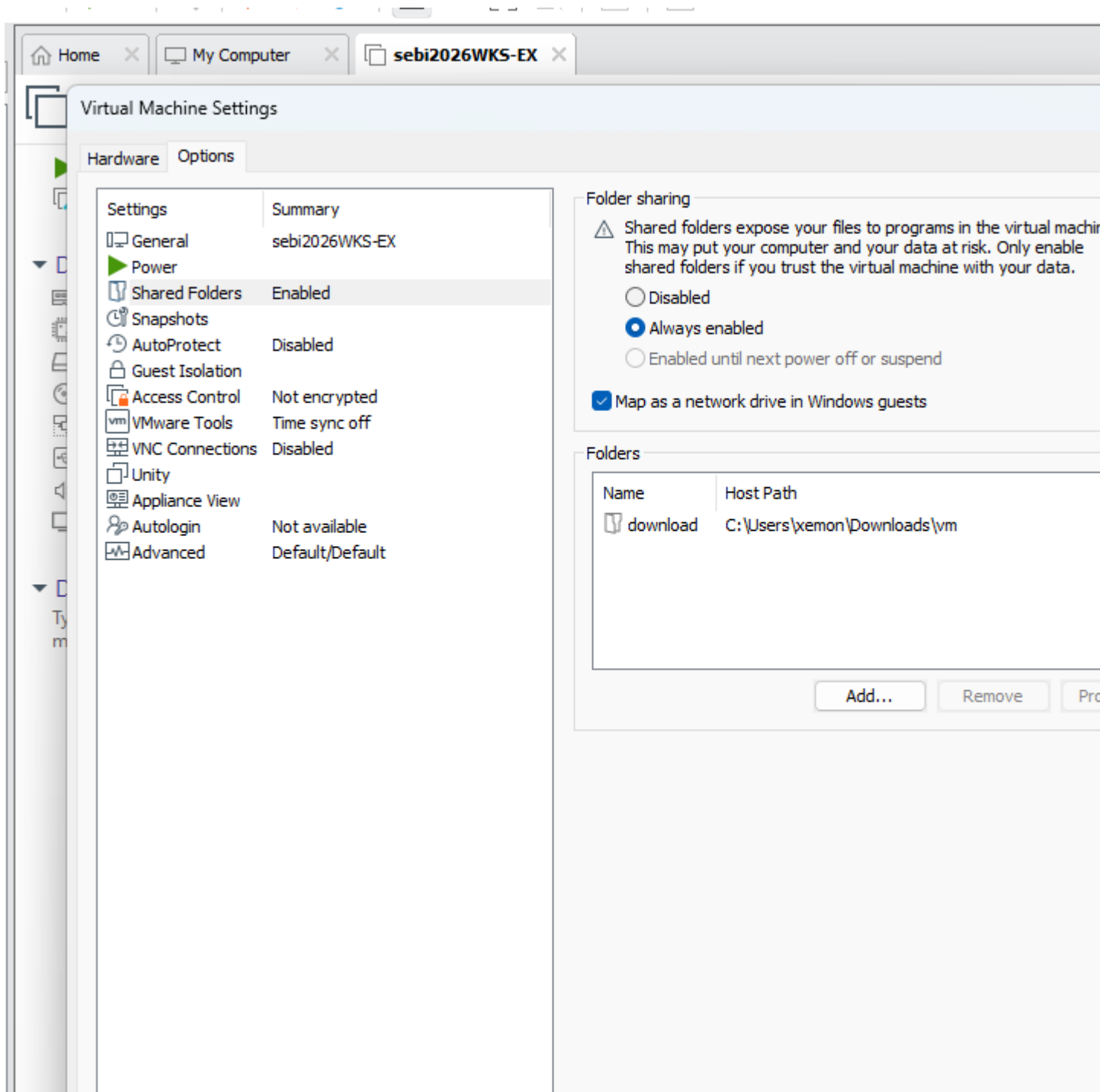
Schermafbeelding 8 — Gedeelde map-instellingen bevestigd voor VM sebi2026WKS-EX
