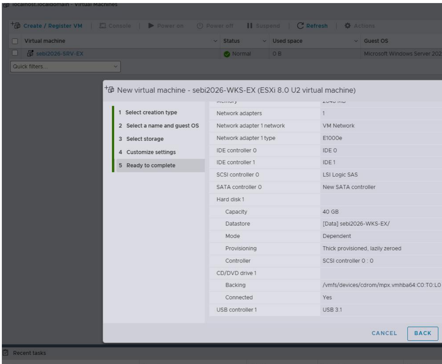
Schermafbeelding 34 — Detail client VM: 40 GB thick provisioned schijf, CD/DVD, USB 3.1 controller
