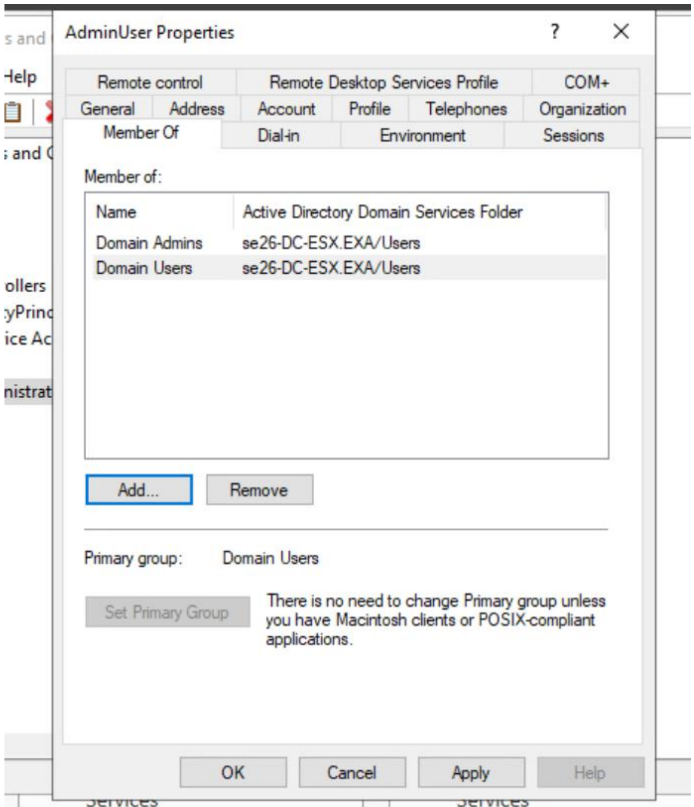
Schermafbeelding 31 — Eigenschappen AdminUser: lid van Domain Admins en Domain Users
