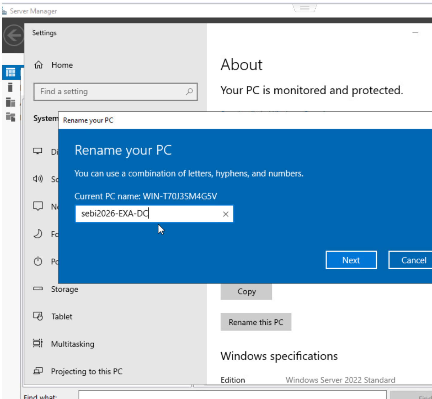
Schermafbeelding 26 — Systeeminstellingen: computernaam gewijzigd naar sebi2026-EXA-DC, Windows Server 2022
