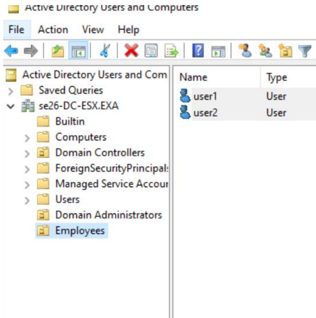
Schermafbeelding 32 — ADUC: domein se26-DC-ESX.EXA met OU's Domain Administrators en Employees, gebruikers user1 en user2
