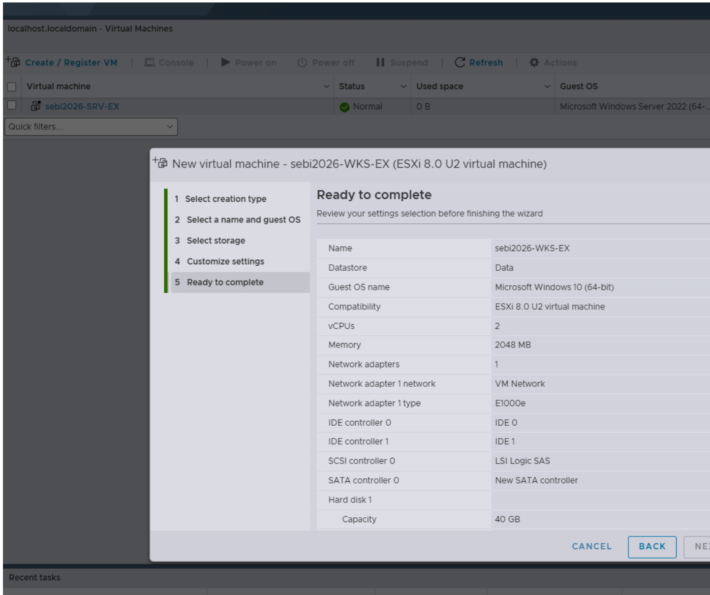
Schermafbeelding 33 — Client VM-instellingen: sebi2026-WKS-EX, 2 vCPU's, 2 GB RAM, 40 GB, E1000e adapter
