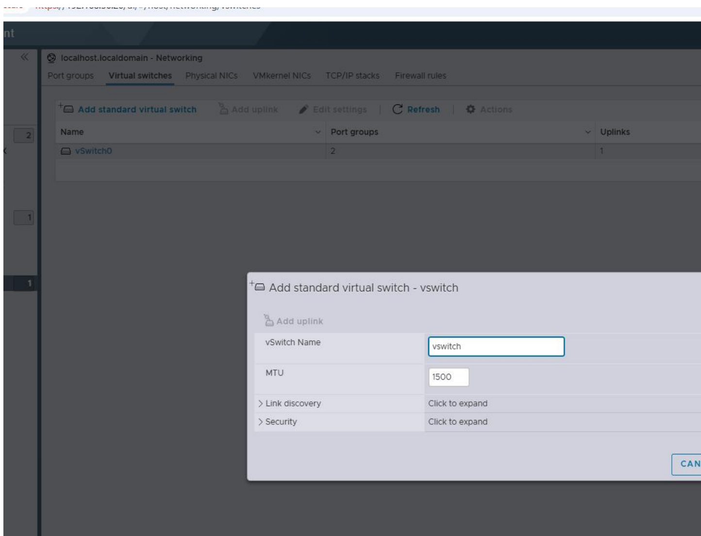
Schermafbeelding 21 — ESXi Netwerken: vSwitch0 met 2 poortgroepen, standaard vSwitch aanmaken
