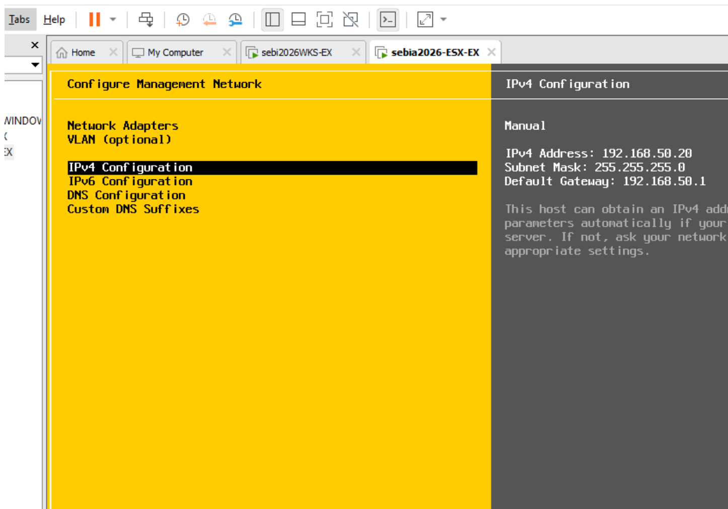
Schermafbeelding 15 — ESXi IPv4-samenvatting: manuele configuratie 192.168.50.20 bevestigd
