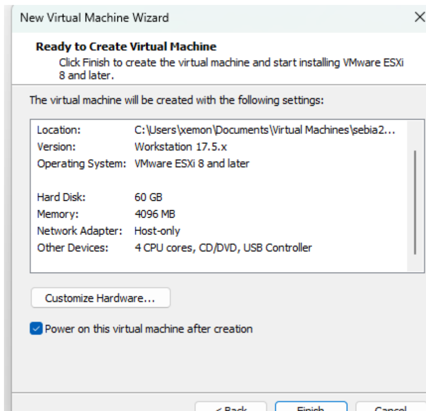
Schermafbeelding 12 — ESXi VM-aanmaak wizard: bevestiging specificaties (overzicht 2)
