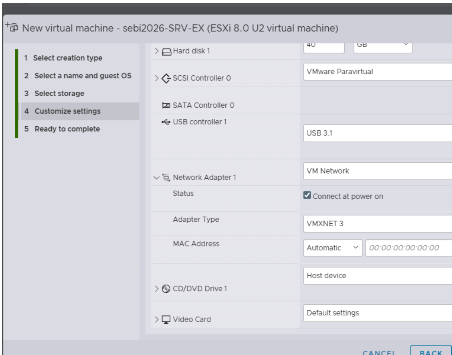
Schermafbeelding 25 — Netwerkinstellingen server VM: VMXNET3, verbinden bij opstarten, automatisch MAC
