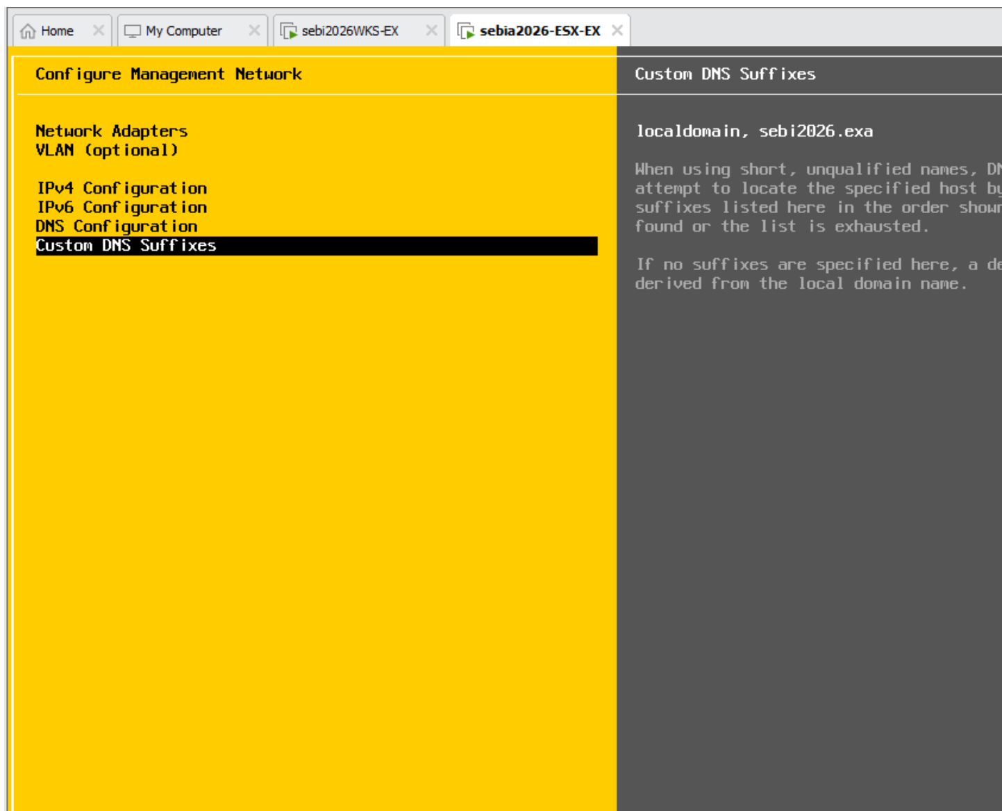
Schermafbeelding 14 — ESXi DNS-achtervoegsel: localdomain en sebi2026.exa ingevoerd
